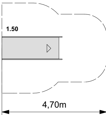
ZRL 9004.150 Breitrutsche 1,50 m Höhe
